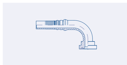
Interlock 90° Swept SAE 3000 PSI (code 61) Flange (SFL 90°)
